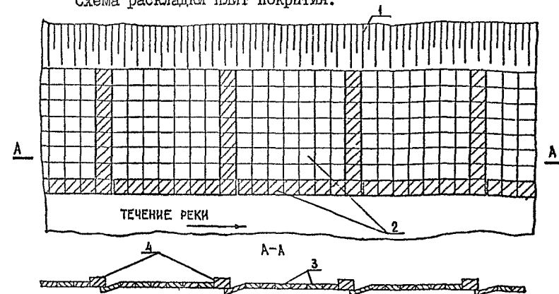
1 – БЕРЕГОВАЯ СТОРОНА; 2 – КАРТЫ ПОКРЫТИЯ; 3 – ЖЕЛЕЗОБЕТОННЫЕ ПЛИТЫ МАССОЙ, РАВНОЙ 0,5 РАСЧЕТНОЙ; 4 – ЖЕЛЕЗОБЕТОННЫЕ ПЛИТЫ РАСЧЕТНОЙ МАССЫ
